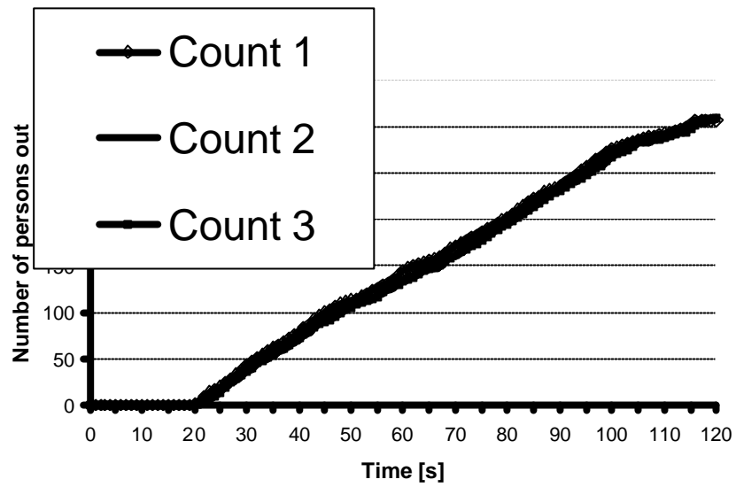
Abbildung 6: Ergebnisse für den Ausgang 2, Erdgeschoss.
