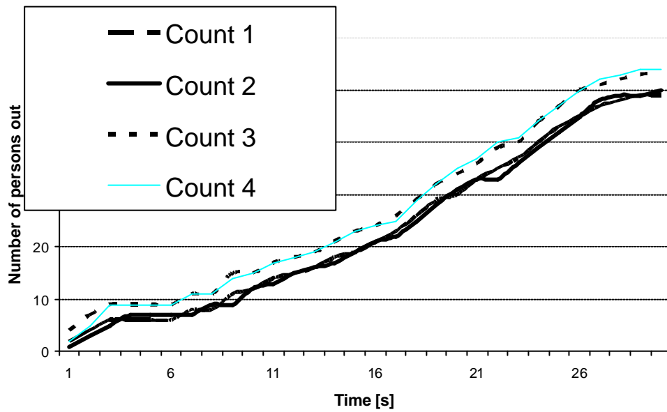
Abbildung 5: Ergebnisse der Übung für den Ausgang 1 Erdgeschoss.
