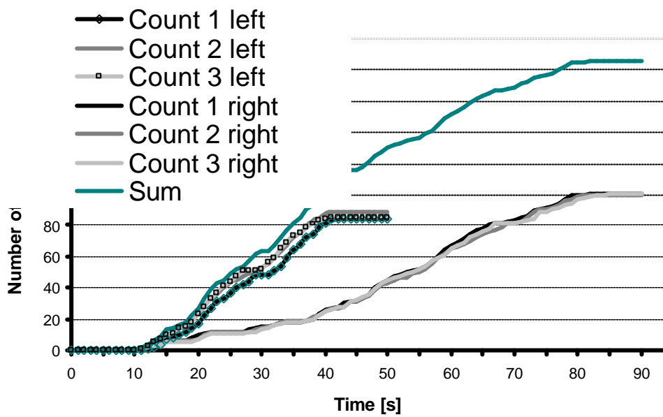
Abbildung 7: Ergebnisse für die Treppe 2. OG der Evakuierungsübung.
